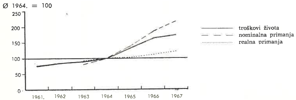
Graf. 6. TROŠKOVI ŽIVOTA, NOMINALNA I REALNA PRIMANJA
